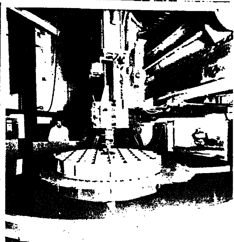
(عين قضائية) جديدة لكبير مرصد فلكي في أوروبا
